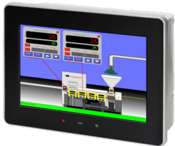
HMI-Bediengeräte in einer Vollaluminium-Konstruktion
