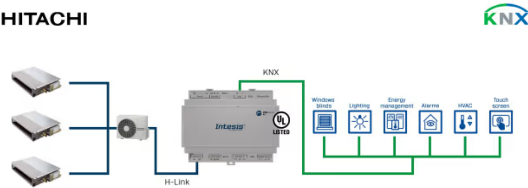
集成示例：使用网关集成 VRF 和 Ait-to-water 系统等混合单元类型时。
